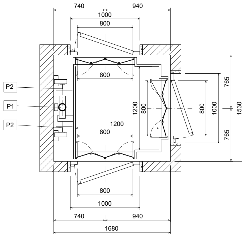
STESSO IMPIANTO INSERITO IN VANO METALLICO : MISURE ESTERNE MONTANTI VANO 1800 x 1630
